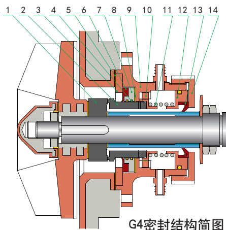
G4密封结构简图
