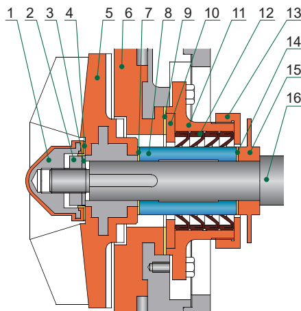
6.1.1 不带冷却水K型动力密封局部图
