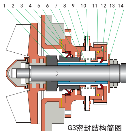
G3密封结构简图
