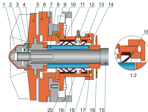
6.1.2 带冷却水K型动力密封局部图
